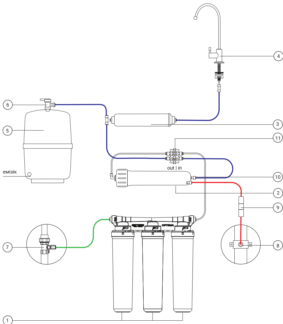
2-сур. Гейзер Престиж/Аллегра Оптима/Гейзер Zero Оптима қосу схемасы
