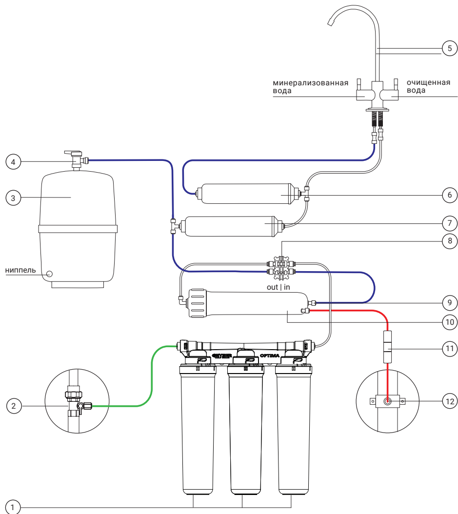
3-сур. Гейзер Zero Оптима М қосу схемасы
