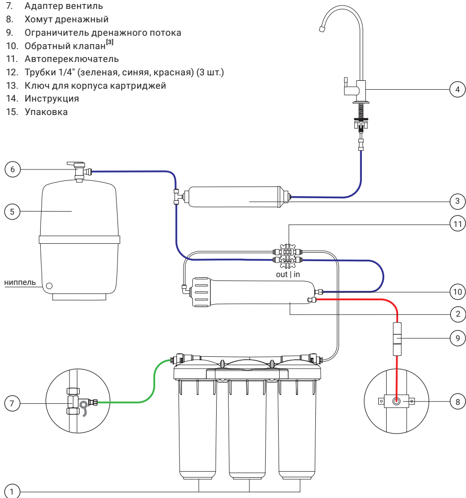
Рис. 2. Схема подключения Гейзер Аллегро/Престиж/Нанотек/Zero 50/Zero 100
